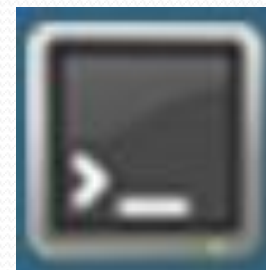
MP3Stego
